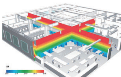
CFDによる室内温熱環境の予測
