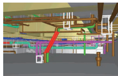
地震時の配管の挙動確認
