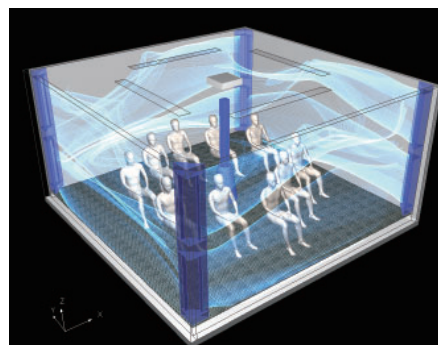
待合エリアの気流分布の再現
