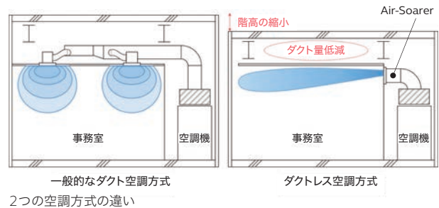
2つの空調方式の違い
