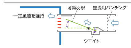
Air-Soarer®の仕組み
